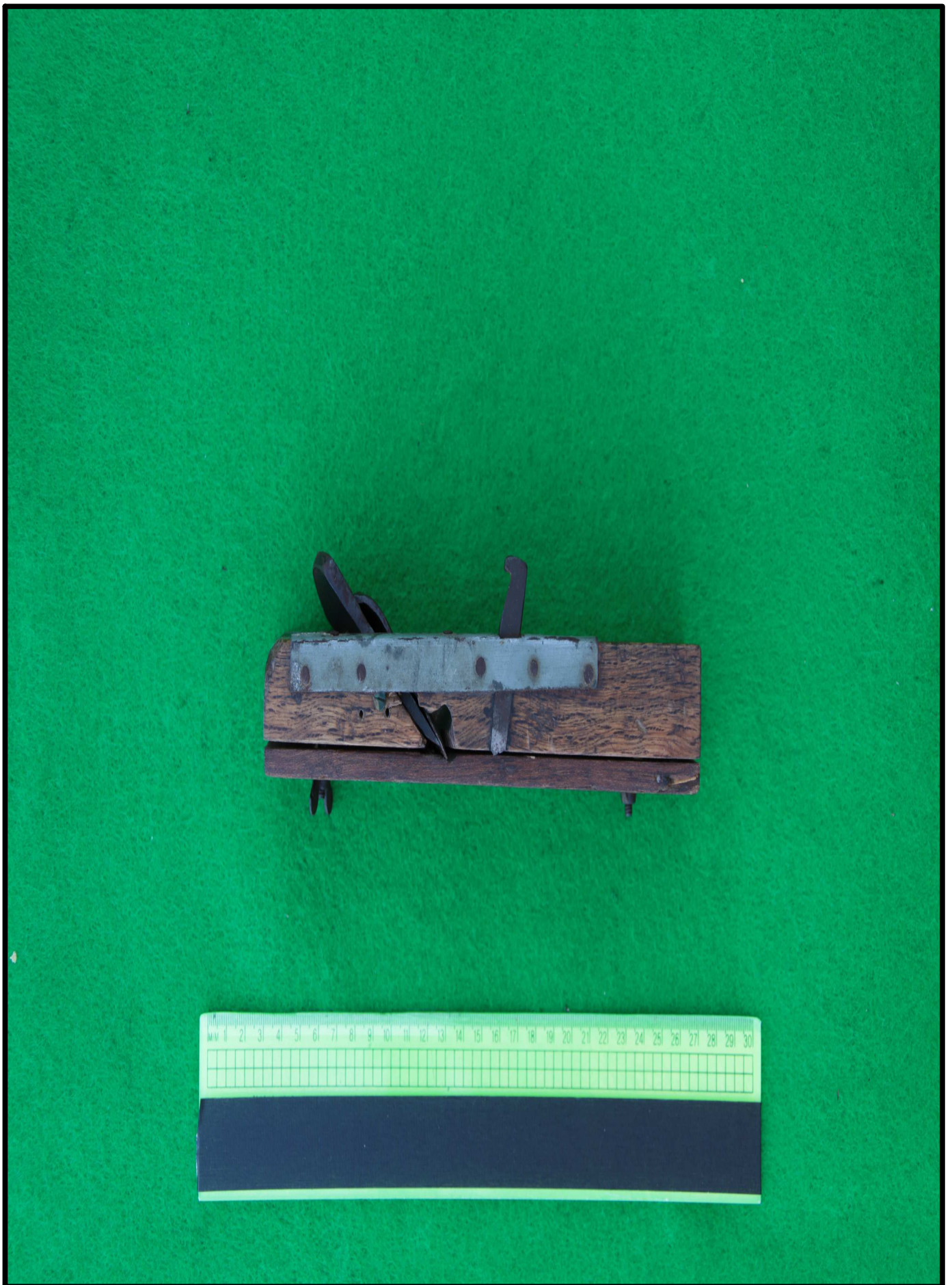
< 모서리대패 옆 >
